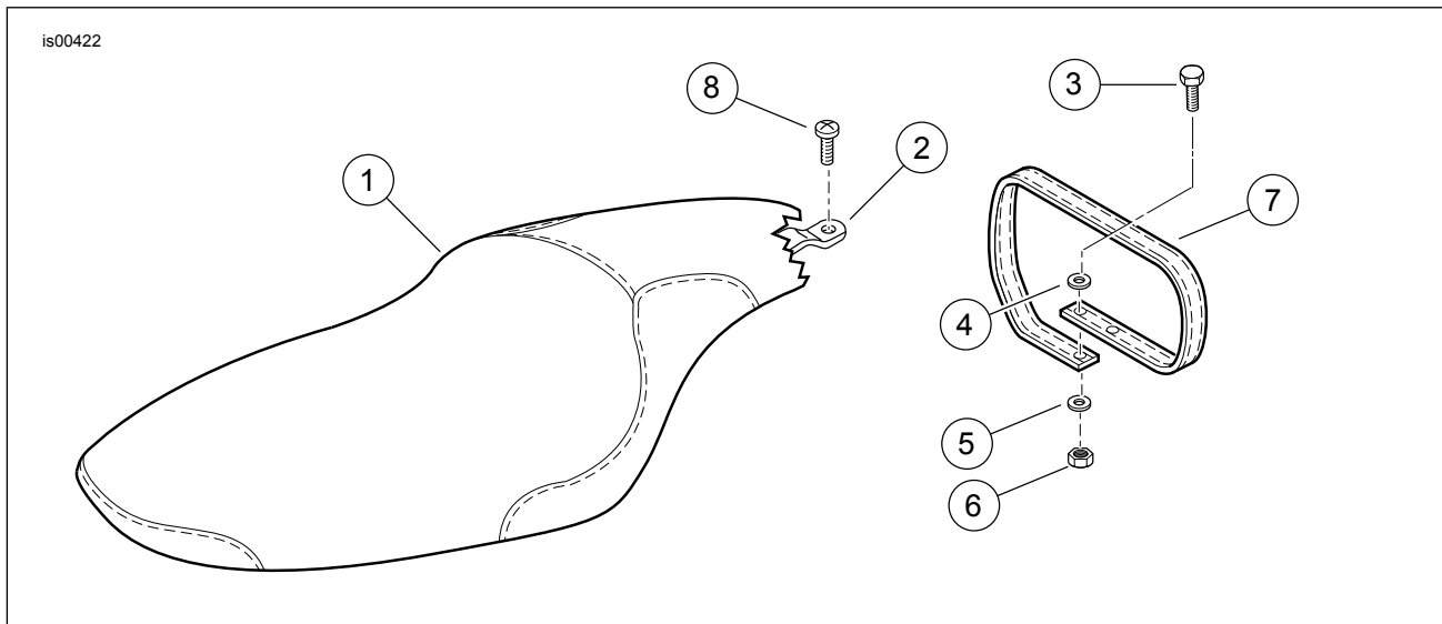
Figura 2. Piezas de servicio: asientos FX Softail
