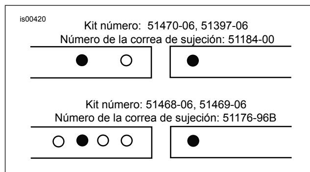
Figura 1. Información de instalación de la correa de sujeción
