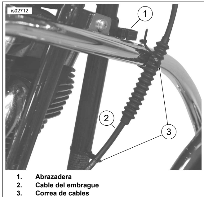
Figura 5. Cable del embrague y correa de cables FXSTD
