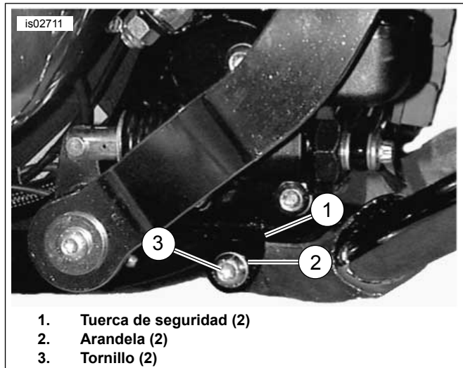
Figura 4. Montaje inferior del protector del motor (visto del lado derecho)
