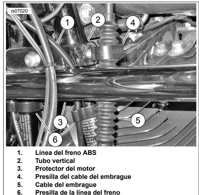
Figura 1. Ubicación del cable del embrague y línea del freno
