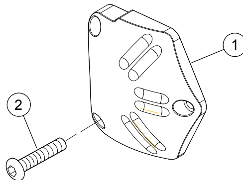
Abbildung 1. Ersatzteile: Magnetschalterabdeckung
