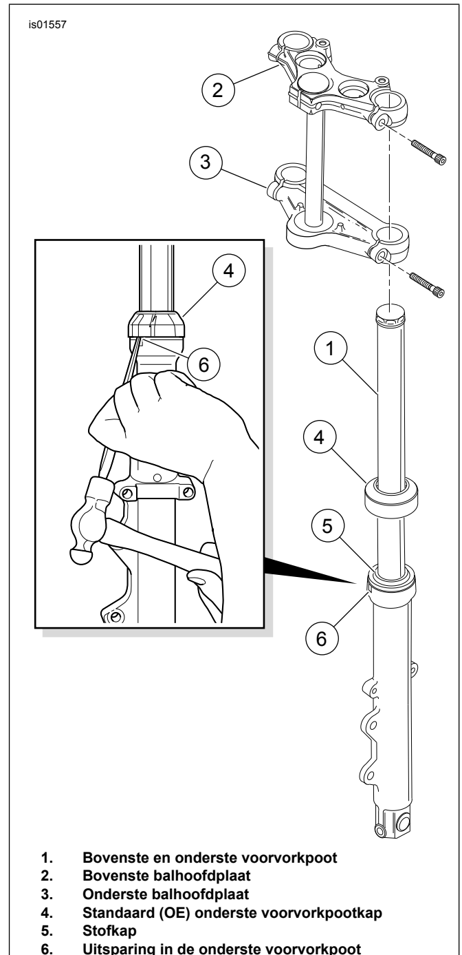
Afbeelding 1. Verwijderen van de onderste voorvorkpootkap
