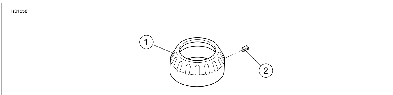
Afbeelding 2. Serviceonderdelen: Kapset (gegolfd) voor onderste voorvorkpoot
