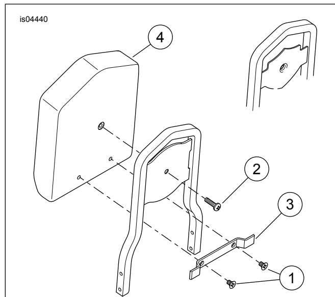
Figura 1. Peças de reposição: Kit do encosto do passageiro
