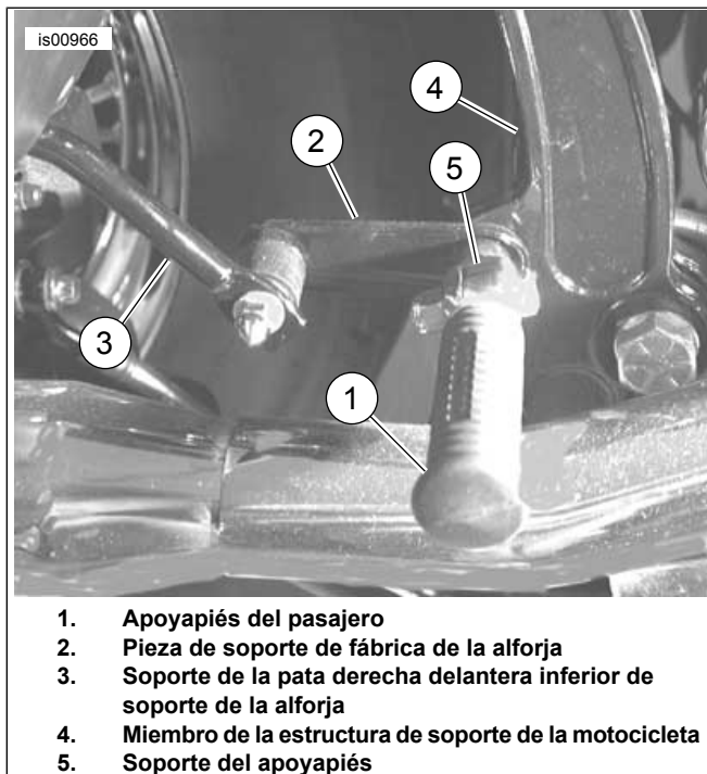
Figura 1. Pieza de soporte de la alforja y apoyapiés del pasajero
