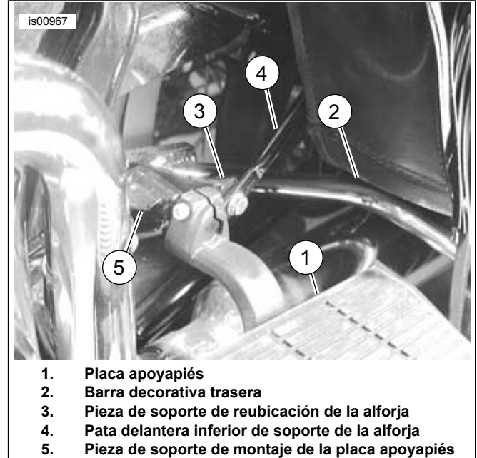
Figura 2. Pieza de soporte de reubicación de la alforja instalada
