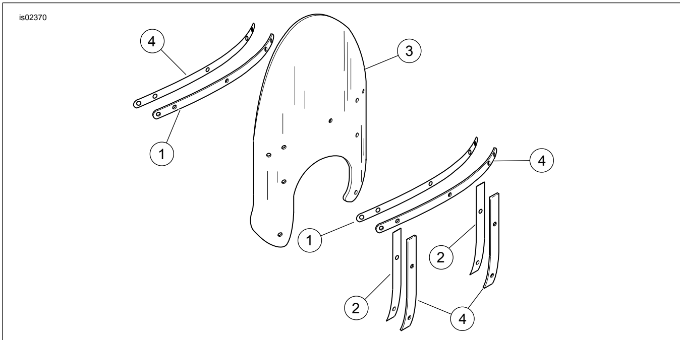
Afbeelding 1. Serviceonderdelen: Windschermsets
