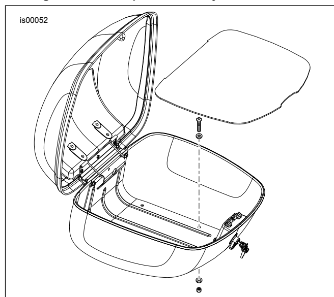
Figura 2. Sujetadores del Tour-Pak
