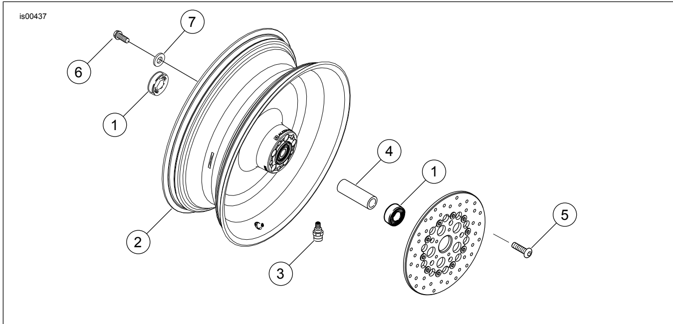
Figura 1. Peças de reposição: kits de roda traseira cromada de 17 pol. (roda com prato sólido mostrada)
