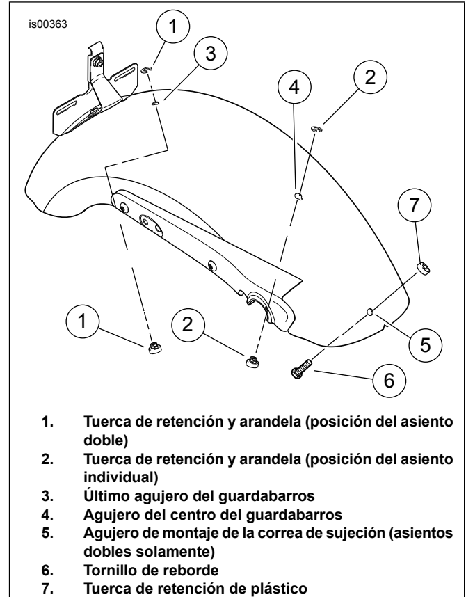
Figura 1. Ubicación de la tuerca de retención
