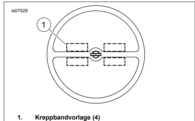
Abbildung 1. Lautsprechergitter
