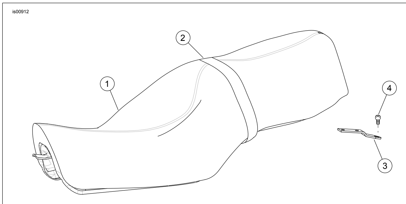
Figure 3. Pièces détachées : siège XL
