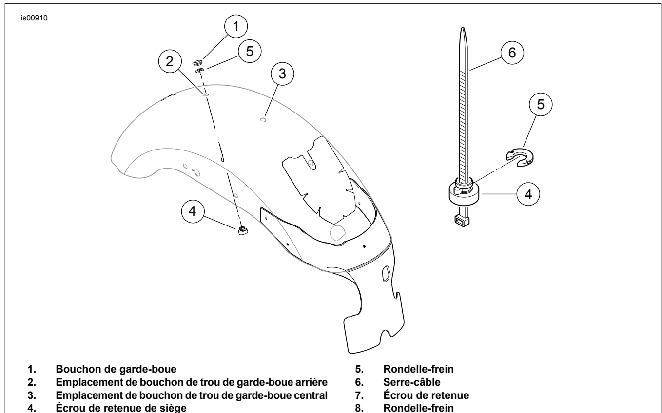
Figure 1. Emplacement des trous de garde-boue
