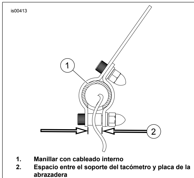
Figura 1. Espacio entre el soporte del tacómetro y placa de la abrazadera
