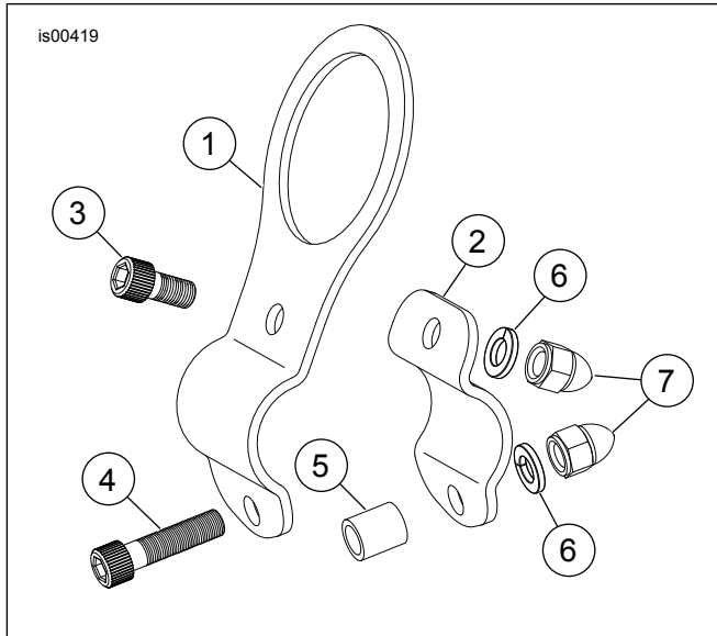
Figura 2. Piezas de servicio para la pieza de soporte del indicador Wide Glide (se muestra la pieza de soporte para indicador sencillo)
