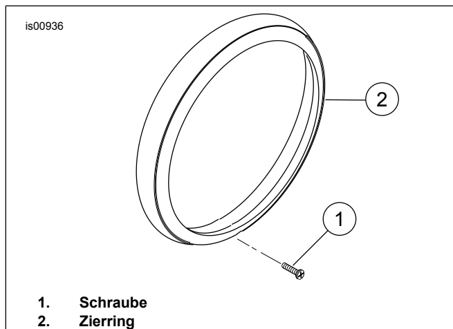
Abbildung 1. Scheinwerfer-Zierring
