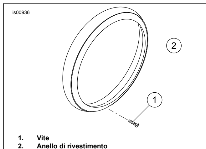
Figura 1. Anello di rivestimento del faro anteriore
