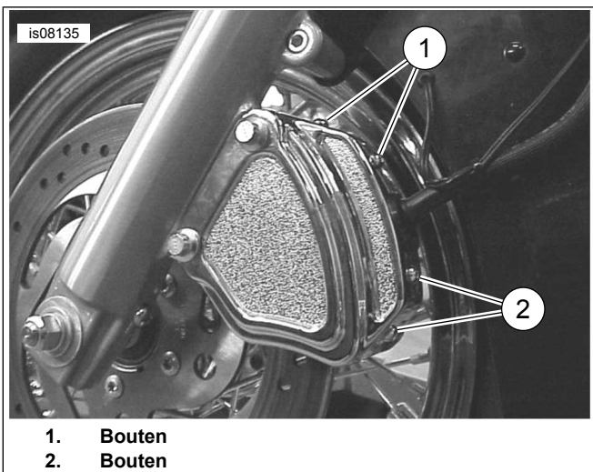
Afbeelding 3. Bouten remklauwkappen monteren
