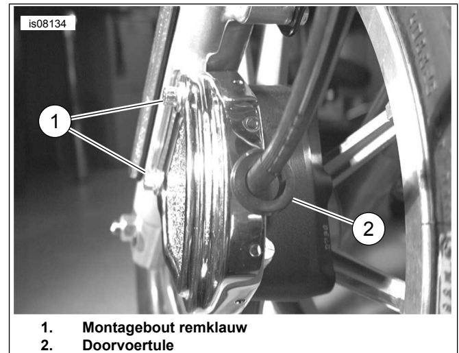
Afbeelding 2. Montagebouten remklauwen vastdraaien en doorvoerrubber monteren
