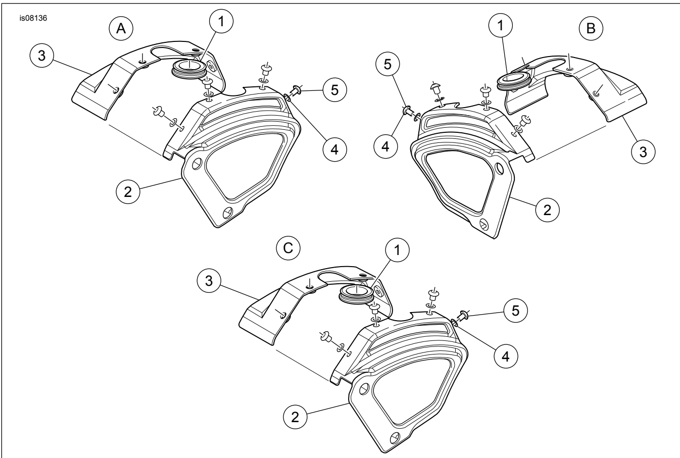
Afbeelding 4. Serviceonderdelen
