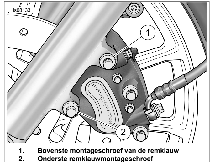
Afbeelding 1. Montagebouten remklauwen verwijderen
