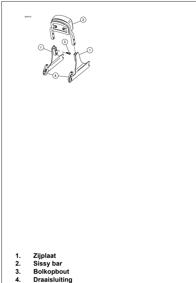
Afbeelding 1. Afneembare sissy bar-zijplaat
