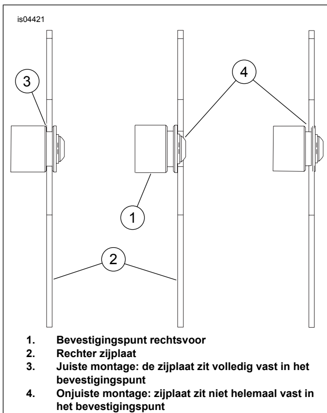
Afbeelding 3. Voorbeelden van juiste/onjuiste montage aan de bevestigingspunten
