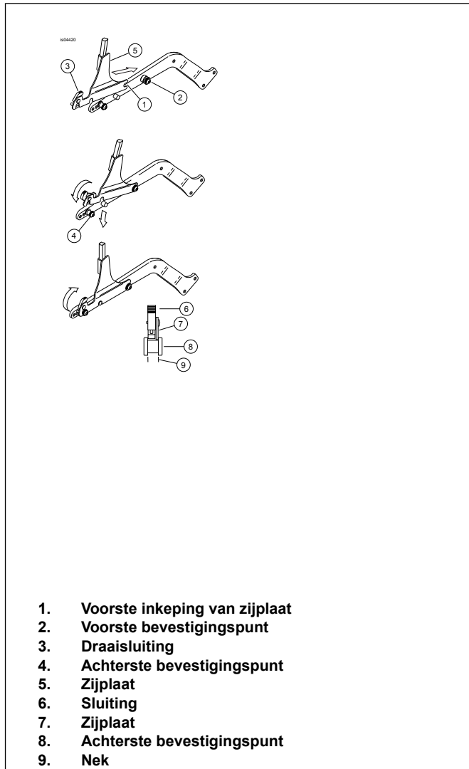
Afbeelding 2. Bevestiging zijplaten sissy bar
