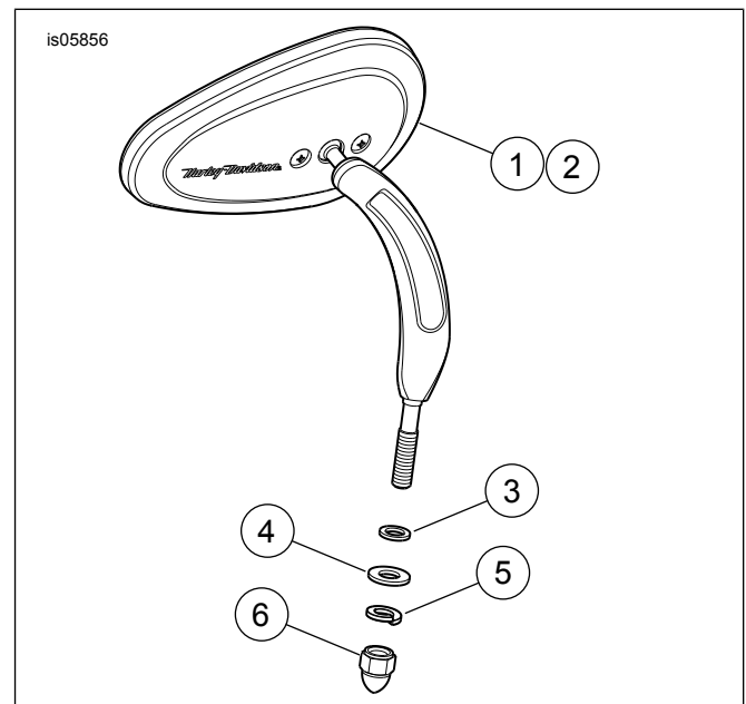
Afbeelding 1. Serviceonderdelen: Spiegelsets (spiegel in Bullet-stijl afgebeeld)
