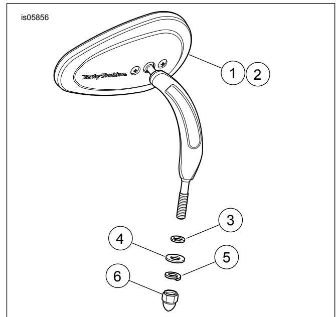
Abbildung 1. Ersatzteile: Spiegelsätze (Zigarrenförmiger Spiegel abgebildet)
