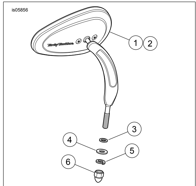
Figura 1. Piezas de servicio: Kits de espejo (se muestra el espejo estilo Bullet)
