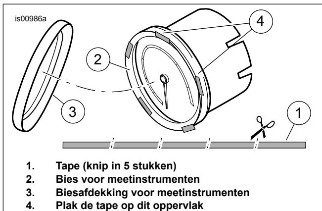
Afbeelding 1. Installeren van de verchroomde instrumentenbies
