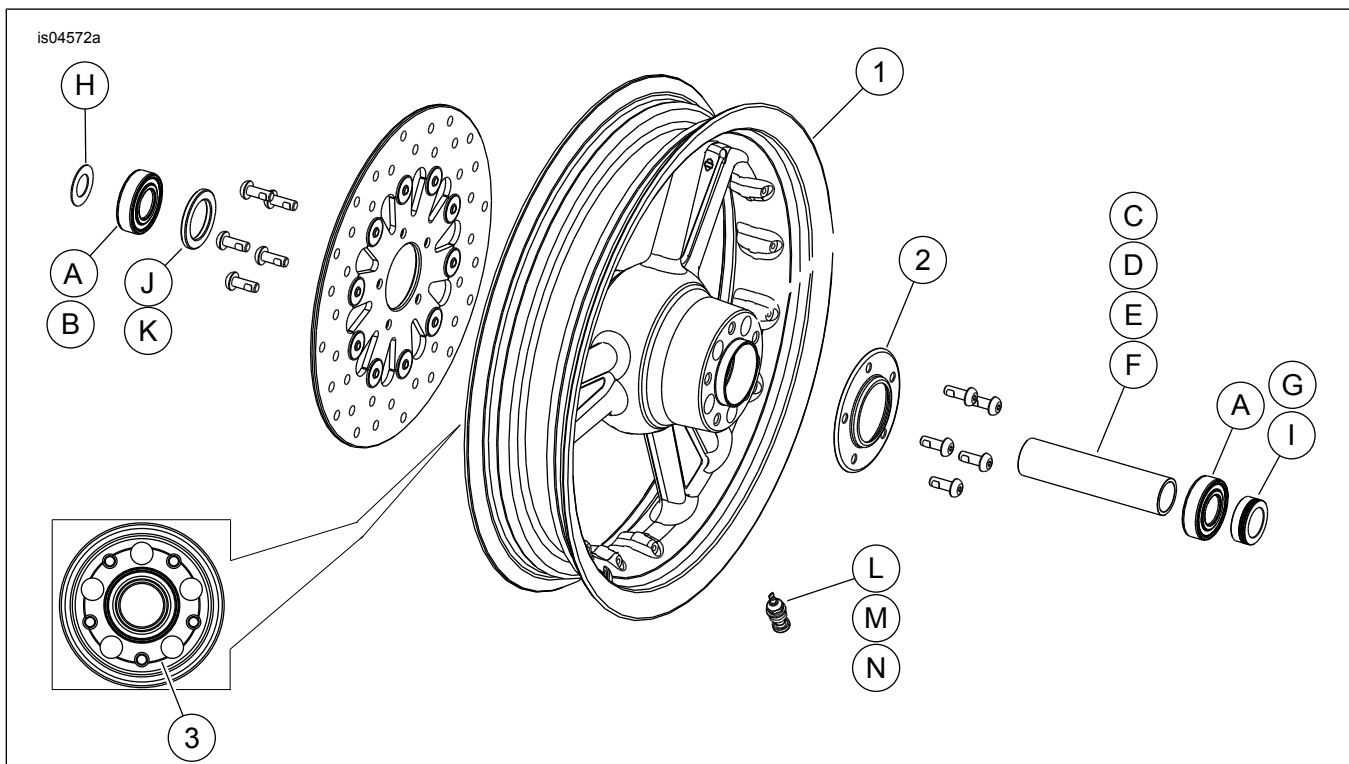
Afbeelding 1. Serviceonderdelen: Detonator voorwielen (16 inch wiel afgebeeld)
