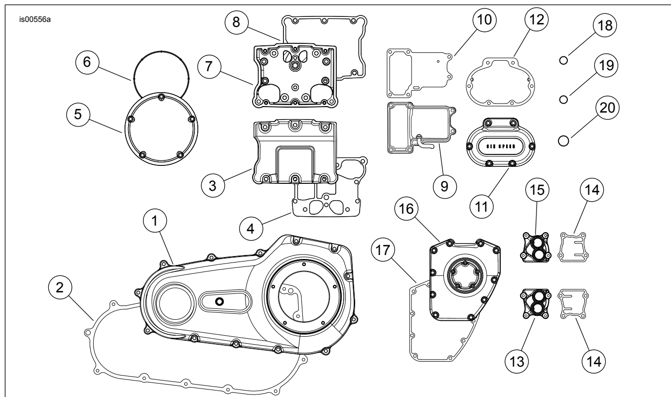
Figura 1. Parti di ricambio, kit coperchio cromato del motore dei modelli Dyna
