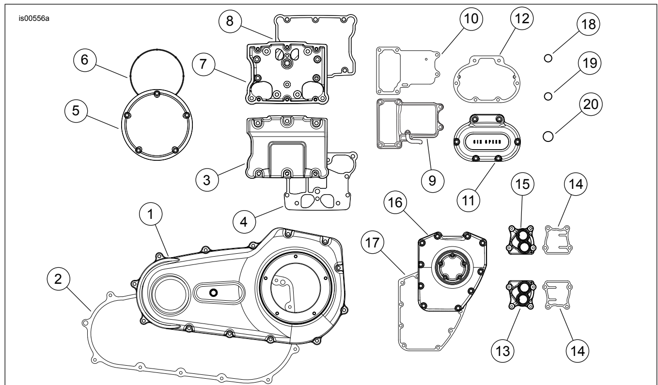
Figura 1. Peças de reposição, kit de tampa cromada do motor Dyna
