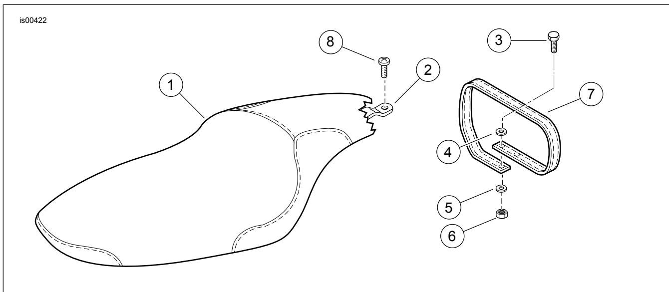
Figura 2. Peças de reposição: assentos da FX Softail
