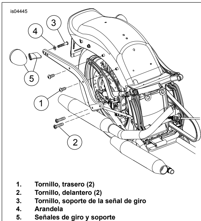
Figura 4. Elementos de sujeción del soporte del guardabarros
