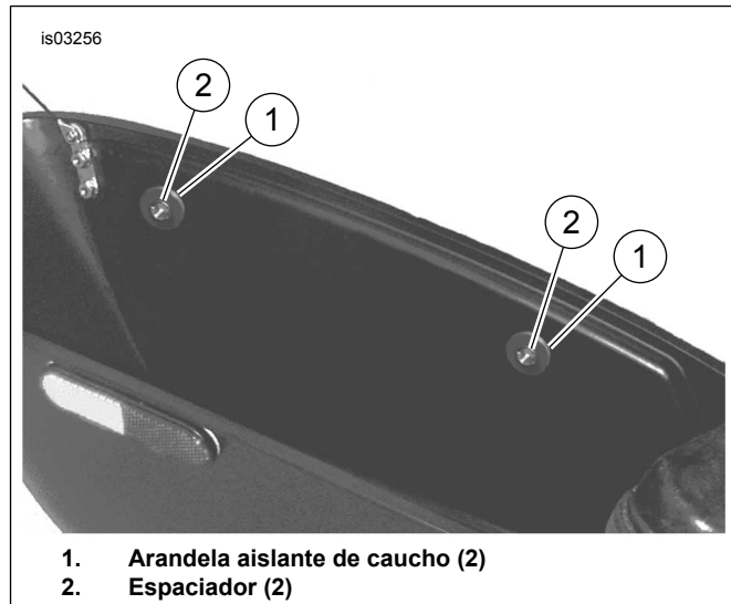
Figura 14. Instalación de las arandelas aislantes y los espaciadores
