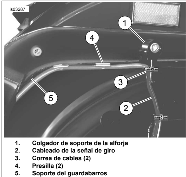
Figura 13. Colocación de cableado e instalación de correas y presillas
