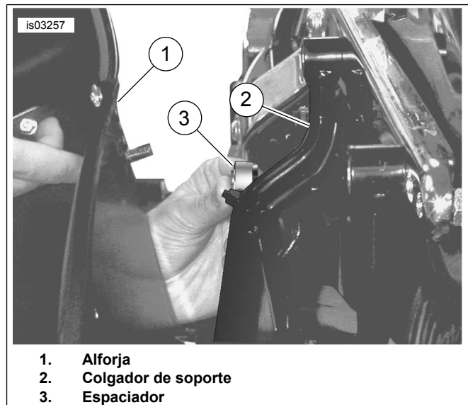
Figura 15. Instalación del espaciador
