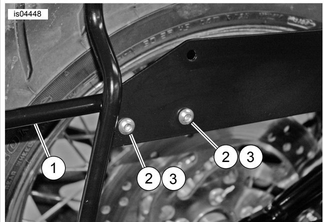
Figura 9. Instalación del colgador de soporte de la alforja
