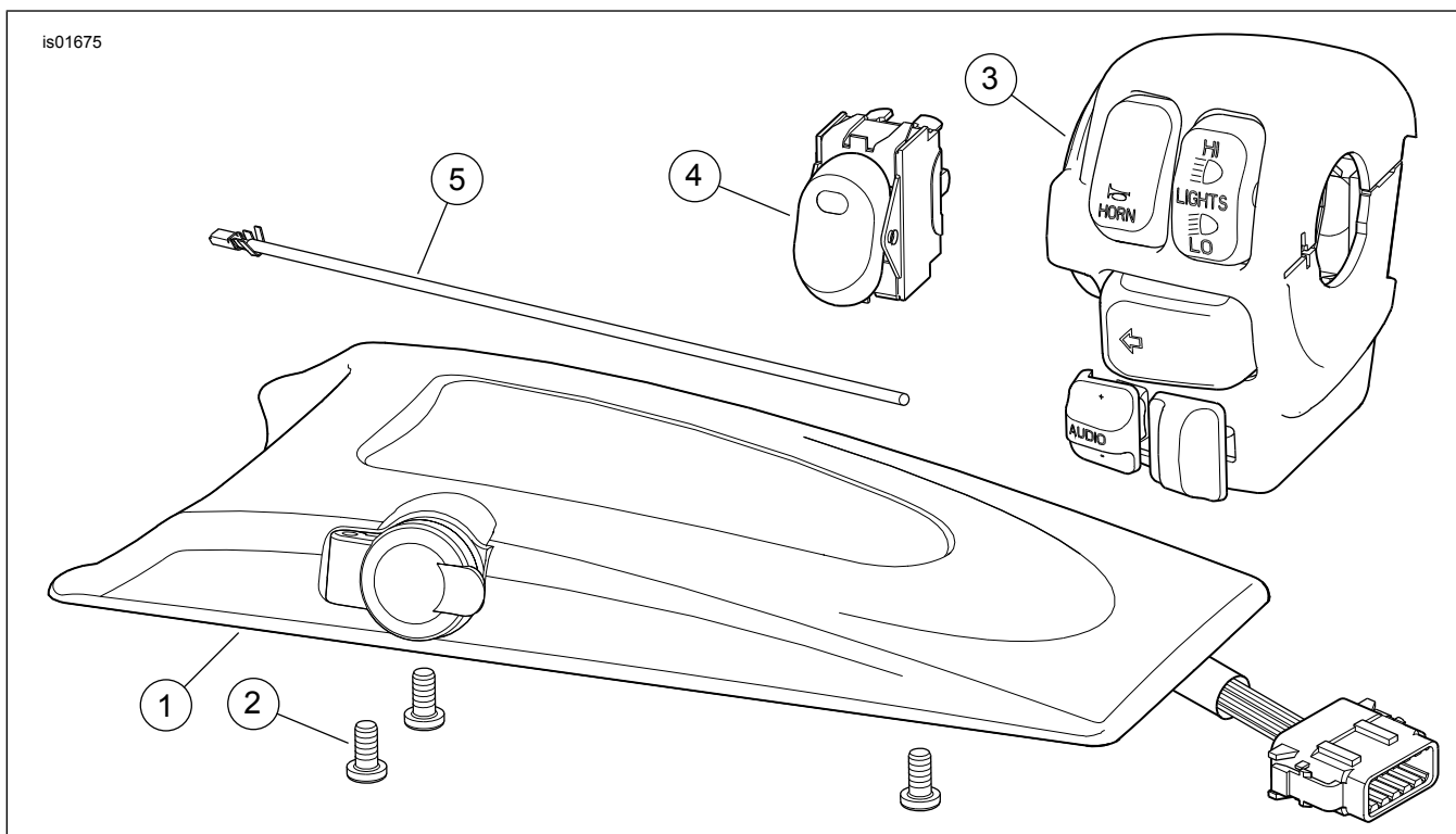
Afbeelding 1. Serviceonderdelen, set 77173-06
