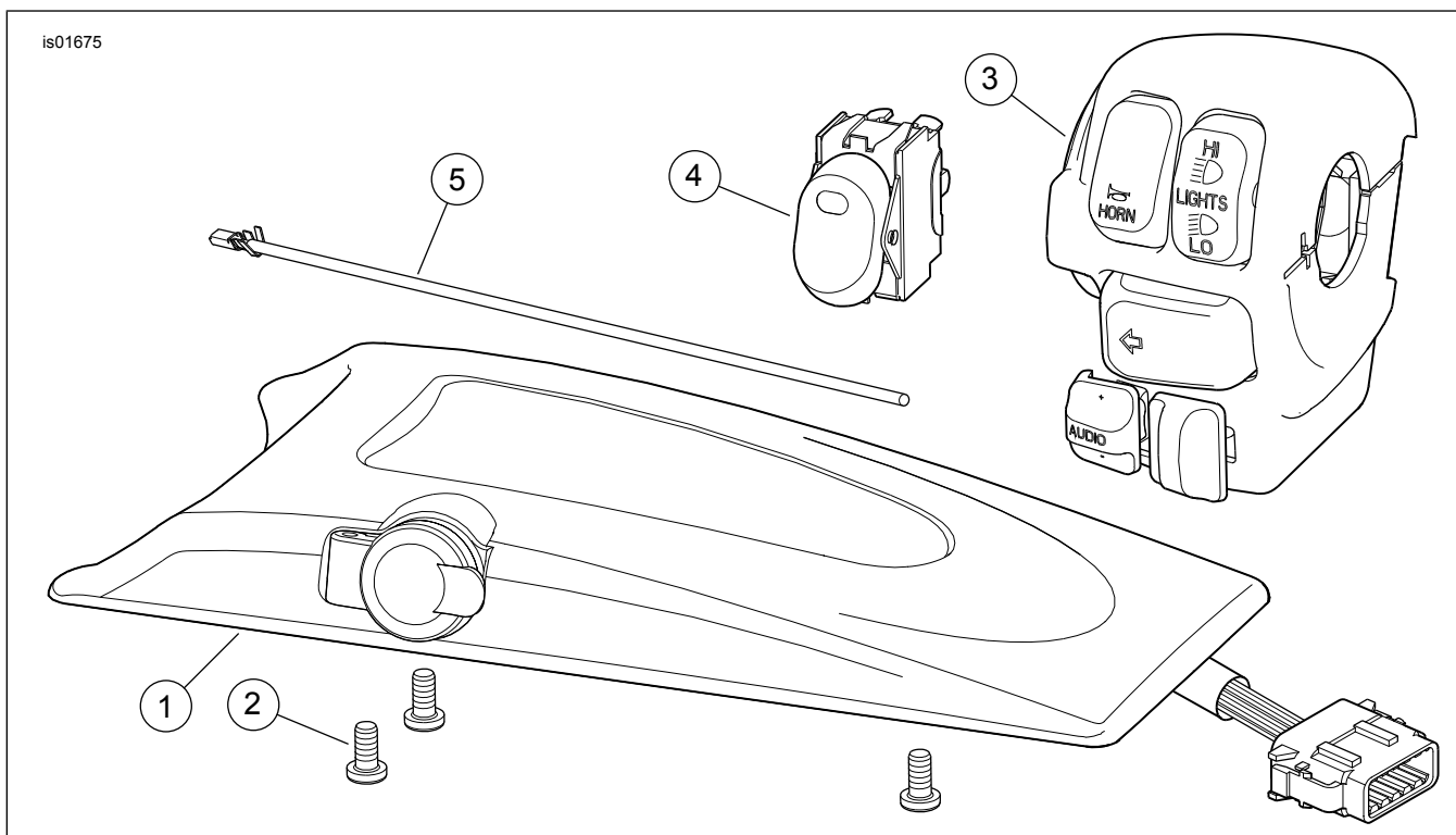
Figura 1. Piezas de servicio: kit 77173-06
