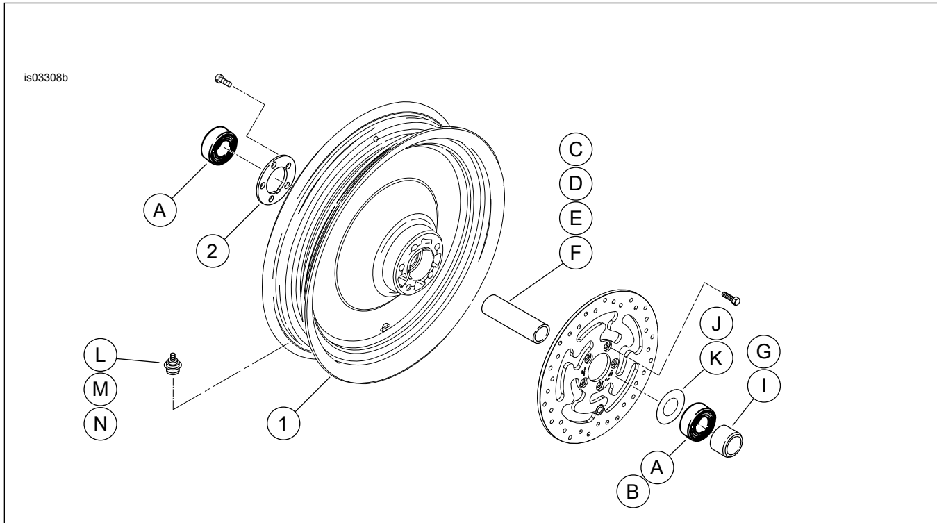
Afbeelding 1. Serviceonderdelen: schijfwielen, voor
