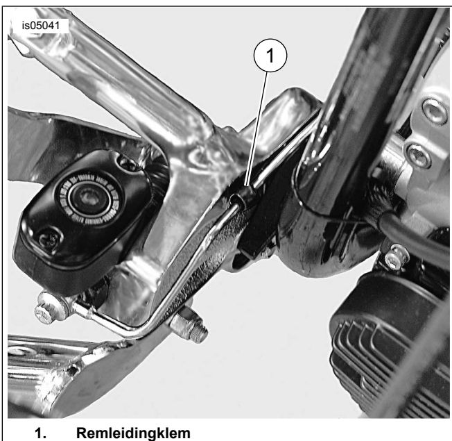
Afbeelding 2. Remleidingklem
