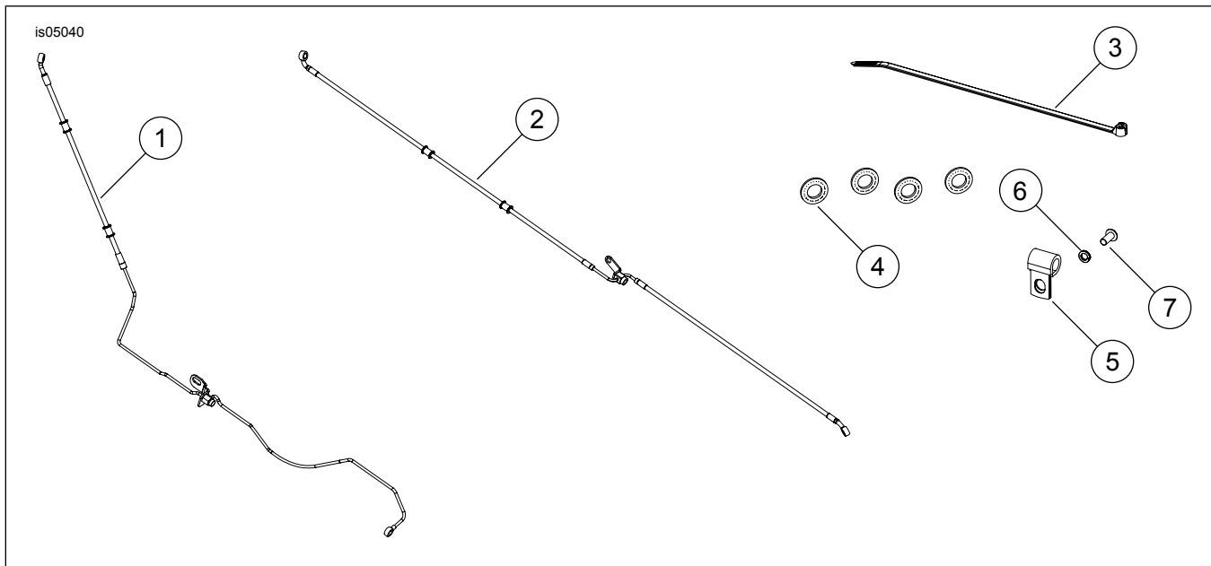
Afbeelding 4. Serviceonderdelen: remleiding voor frontbesturing met verlengd bereik
