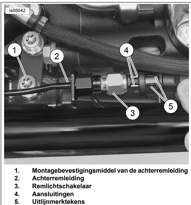
Afbeelding 1. Remleidingsteun en remlichtschakelaar
