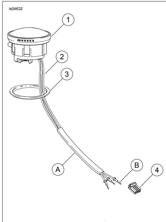
Figura 2. Piezas de servicio: kit de indicador LED de combustible
