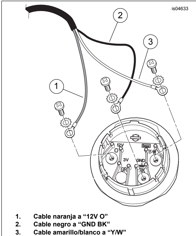
Figura 1. Conexiones de los cables
