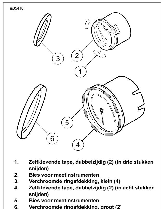
Afbeelding 1. Instrumentringen installeren
