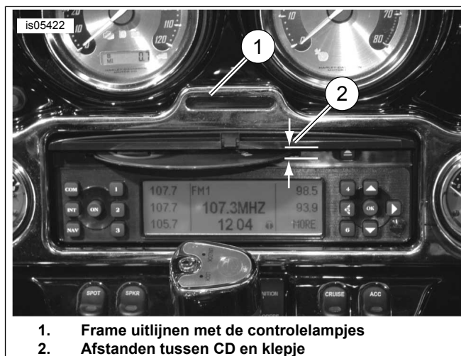
Afbeelding 4. Radio-/meterring installeren
