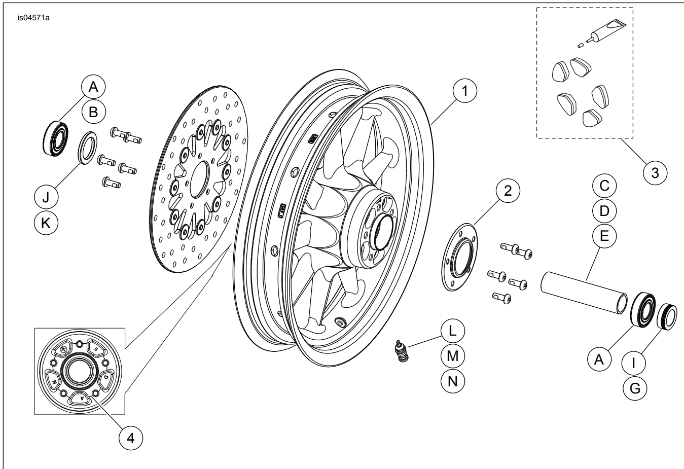
Afbeelding 1. Servicehandleiding: Negenspaaks voorwielen
