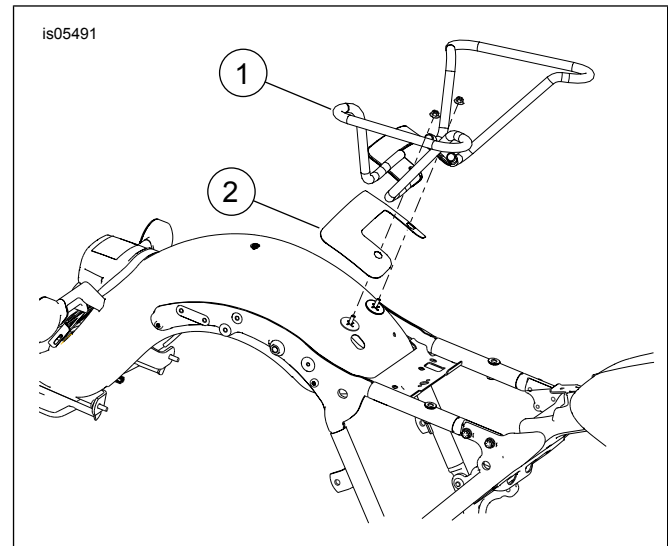
Abbildung 1. Ersatzteile: Soziushaltebügel
