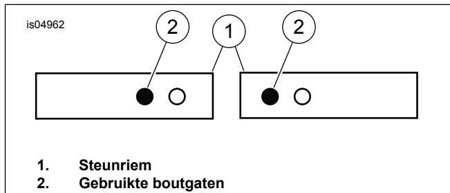
Afbeelding 3. Configuratie steunriem
