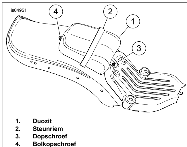
Afbeelding 4. Installeren van de duozit
