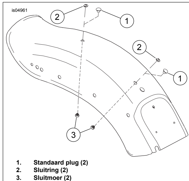
Afbeelding 1. Verwijderen van de plug en installeren van de sluitmoer
