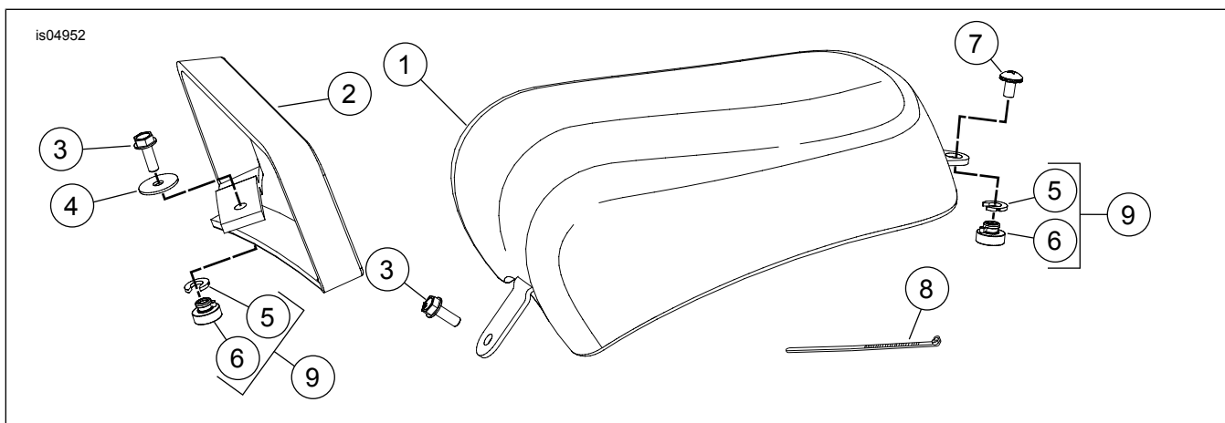
Afbeelding 5. Serviceonderdelen voor FLSTSB-duozit
