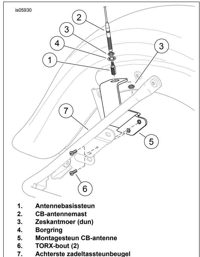
Afbeelding 3. Bevestigen van de montagesteun van de CB-antenne aan het spatbord
