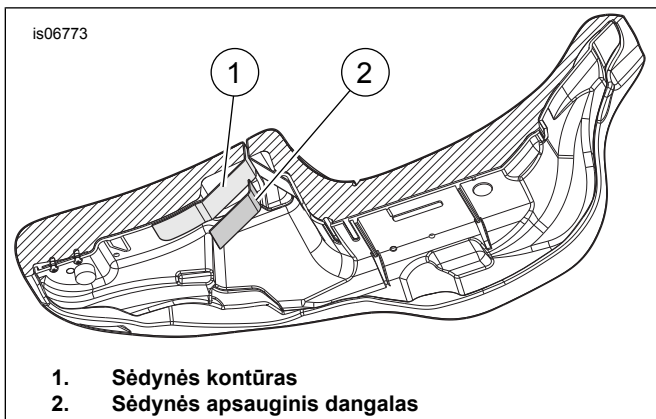
Pav 9. Sėdynės apatinė pusė
