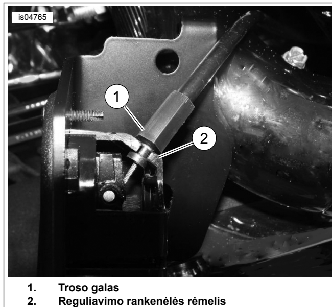
Pav 7. Sėdynės reguliavimo trosas padėtis (vaizdas iš taško po sumontuota rankenėle)
