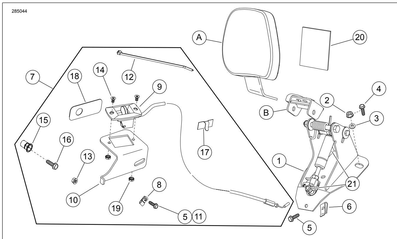
Pav 14. Dalys, reikalingos užduočiai atlikti Motociklininko reguliuojamo atlošo montavimo detalių kompleksas
