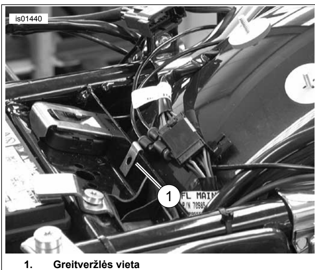
Pav 4. Greitveržlės montavimas
