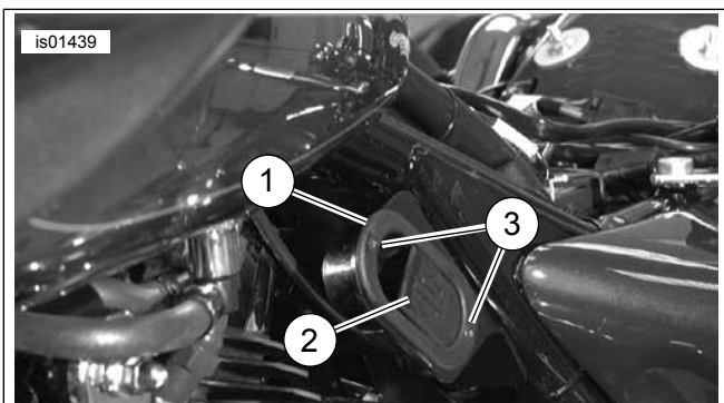
1. Reguliavimo rankenėlės rėmelis (parodytas įprastinis) 2. Atlošo reguliavimo rankenėlė 3. Varžtas (2)
