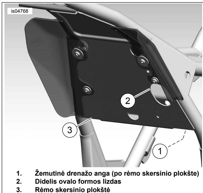
Pav 8. Atlošo trosų vedimas per rėmą (pavaizduoti 2008 m. modeliai)
