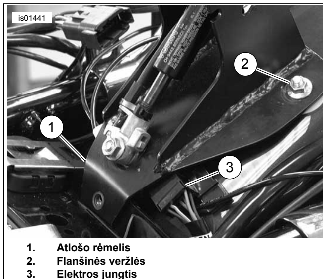
Pav 6. Atlošo rėmelio tvirtinimas naudojant flanšines veržles ir sraigta
