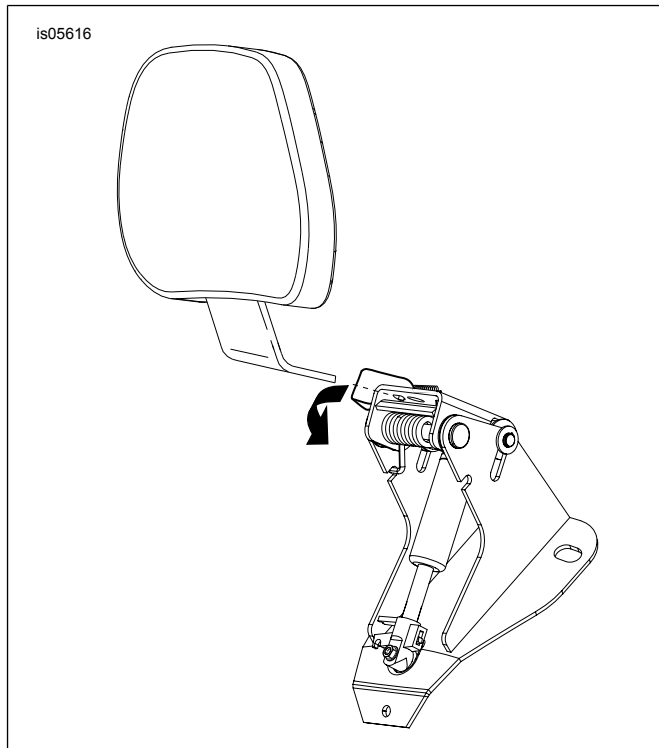
Pav 12. Atlošo montavimas
