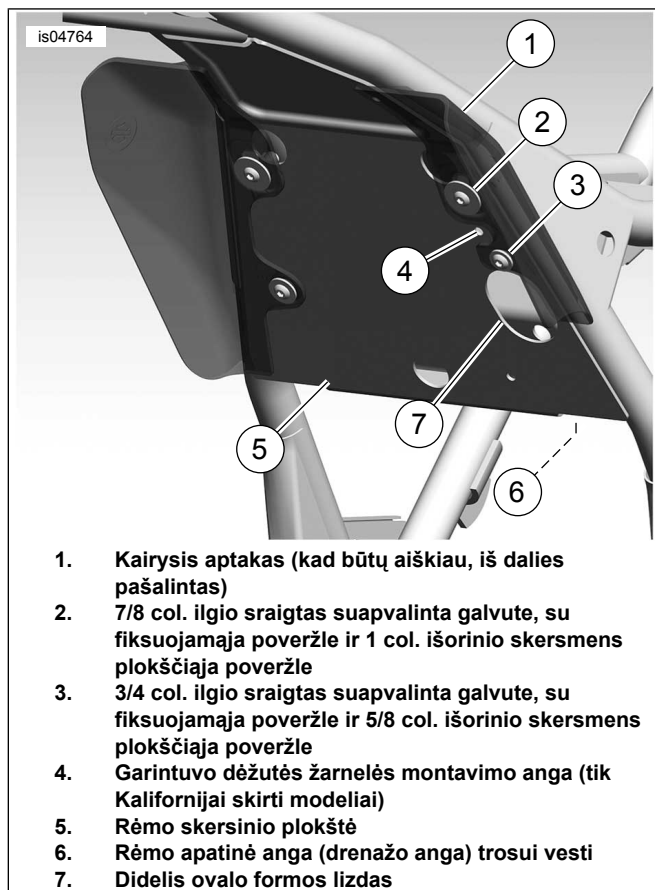
Pav 5. 2008 m. modeliai: tvirtinimo elementų vietos – rėmo vaizdas žiūrint link užpakalio nuo užpakalinio cilindro (kad būtų aiškiau, variklis pašalintas)
