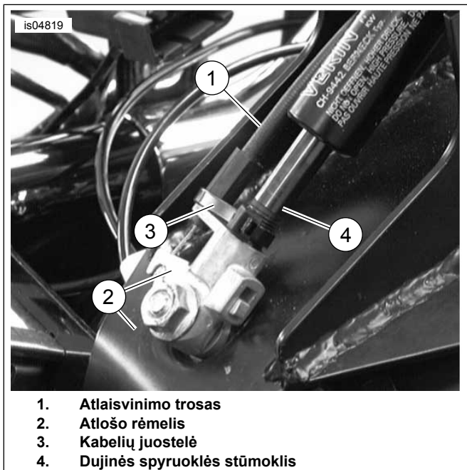
Pav 11. Trosio tvirtinimas prie atlošo rėmelio
