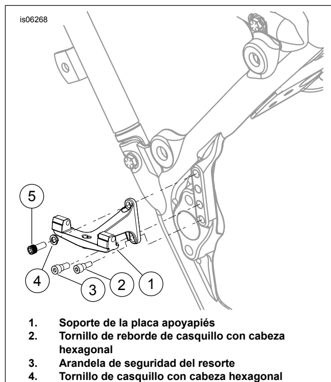
Figura 1. Instalación del soporte de la placa apoyapiés
