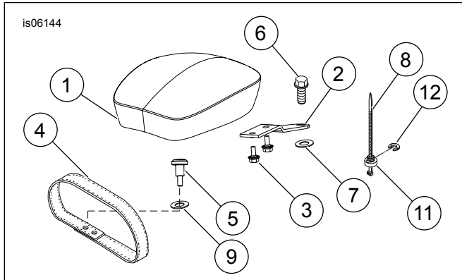
Afbeelding 2. Serviceonderdelen: XL-passagierskussen
