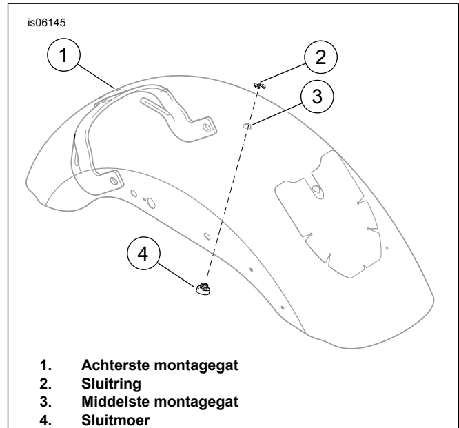
Afbeelding 1. Montagegaten in spatbord
