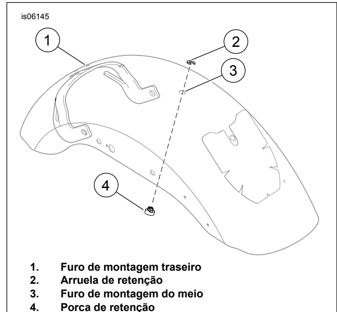
Figura 1. Furos de montagem do para-lama
