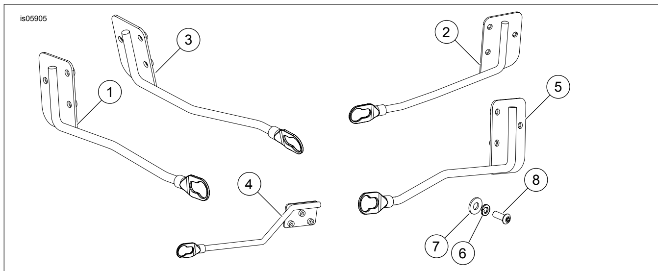
Afbeelding 1. Serviceonderdelen: onderste steunbeugelset voor afneembare zadeltas
