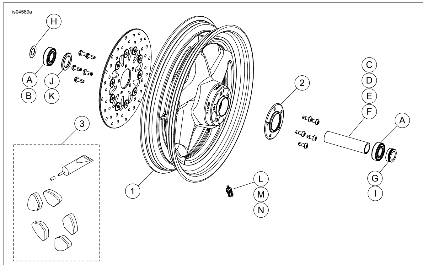
Afbeelding 2. Reaper voorwiel (21 inch wiel afgebeeld)
