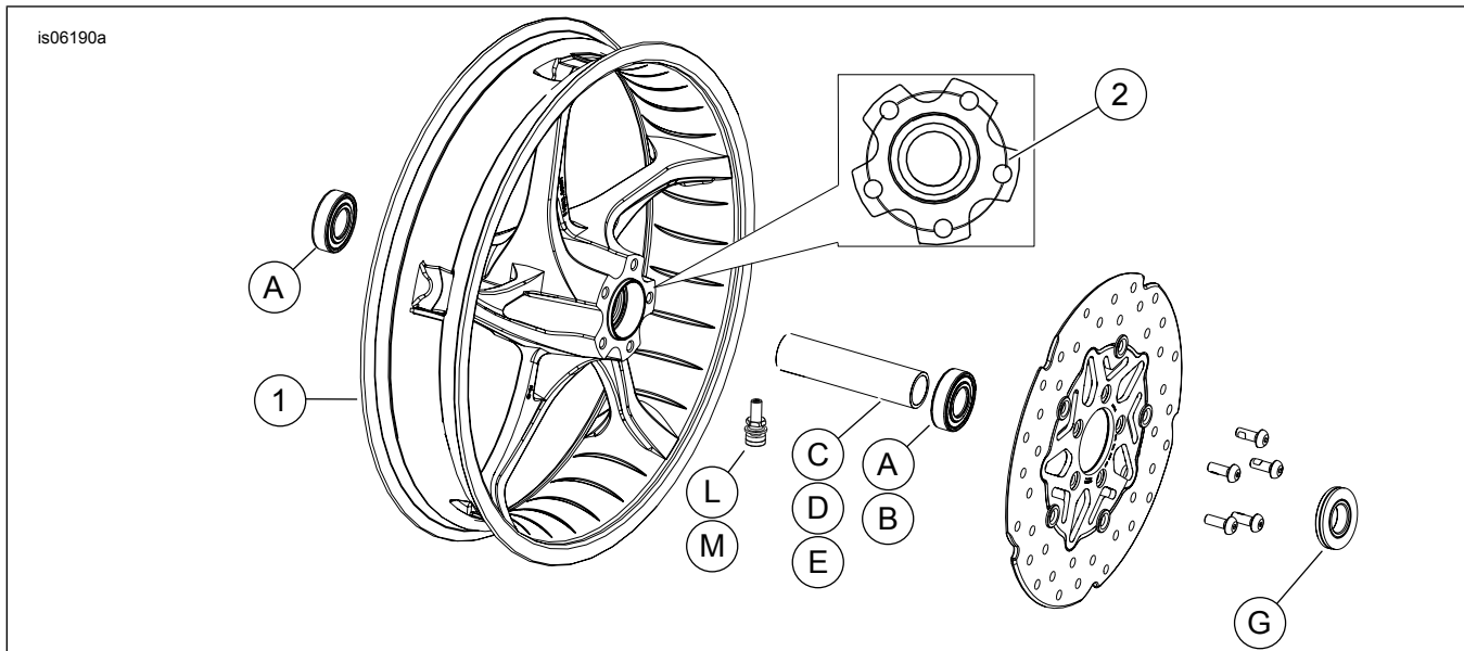
Afbeelding 1. Serviceonderdelen: Voorwiel, Stinger
