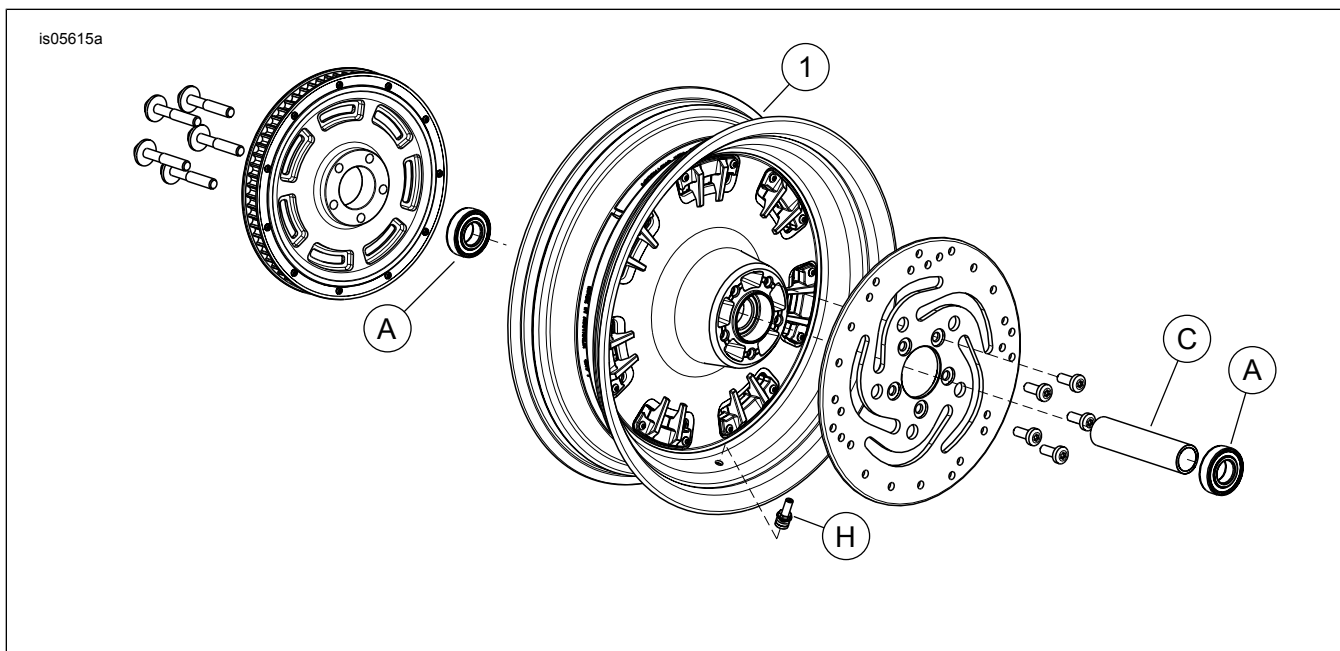
Afbeelding 1. Serviceonderdelen: Fang-achterwiel
