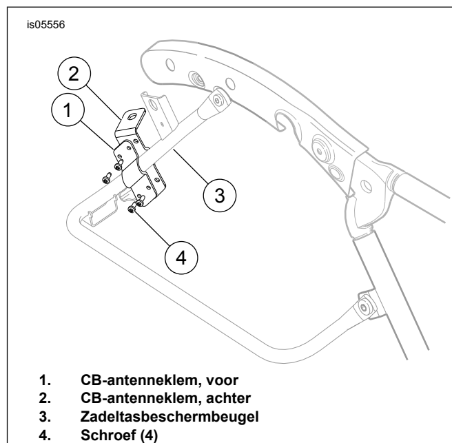
Afbeelding 1. Plaats van de bevestigingssteun van de antenne
