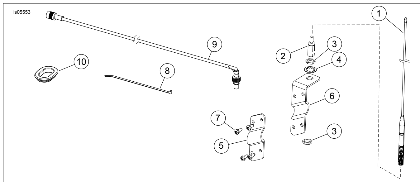
Afbeelding 2. Serviceonderdelen: CB-antenne voor montage op het frame
