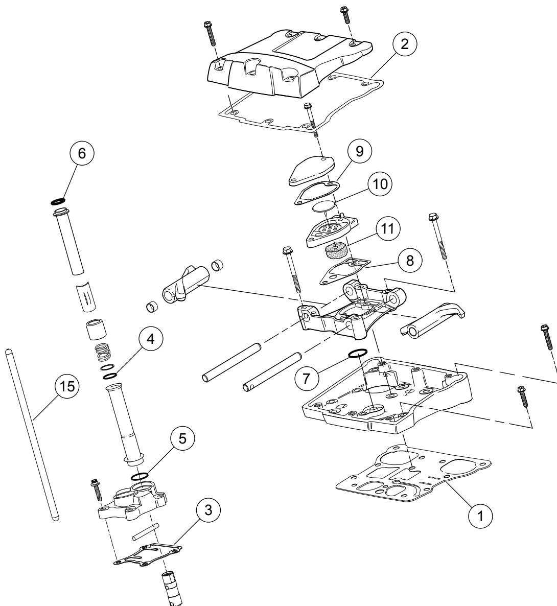
Afbeelding 2. Serviceonderdelen: Screamin' Eagle Pro TC 1690 cm³ (103 in³) Stage 3-set
