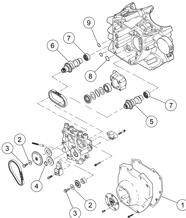
Afbeelding 3. Serviceonderdelen: Screamin' Eagle Pro TC 1690 cm 3 (103 in 3 ) Stage 3-set
