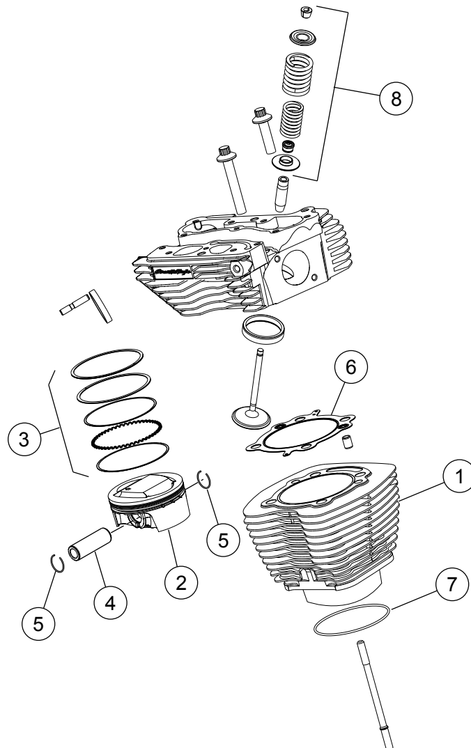
Afbeelding 1. Serviceonderdelen: Screamin' Eagle Pro TC 1690 cm³ (103 in³) Stage 3-set
