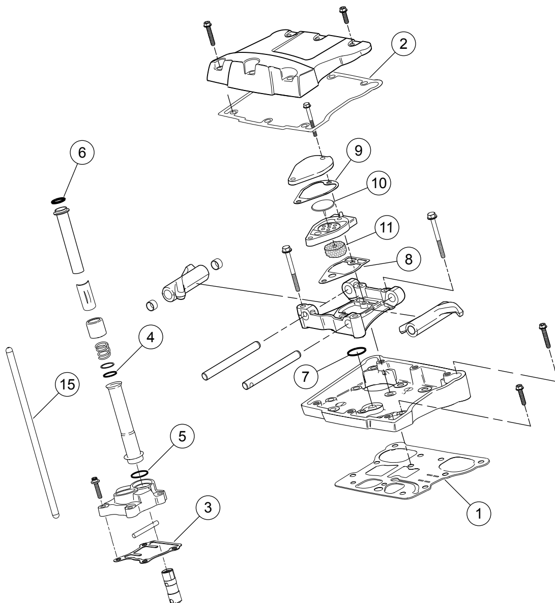
Figura 2. Parti di ricambio: Kit Stage 3 Screamin' Eagle Pro TC 1.690 cm 3 (103 in 3 )
