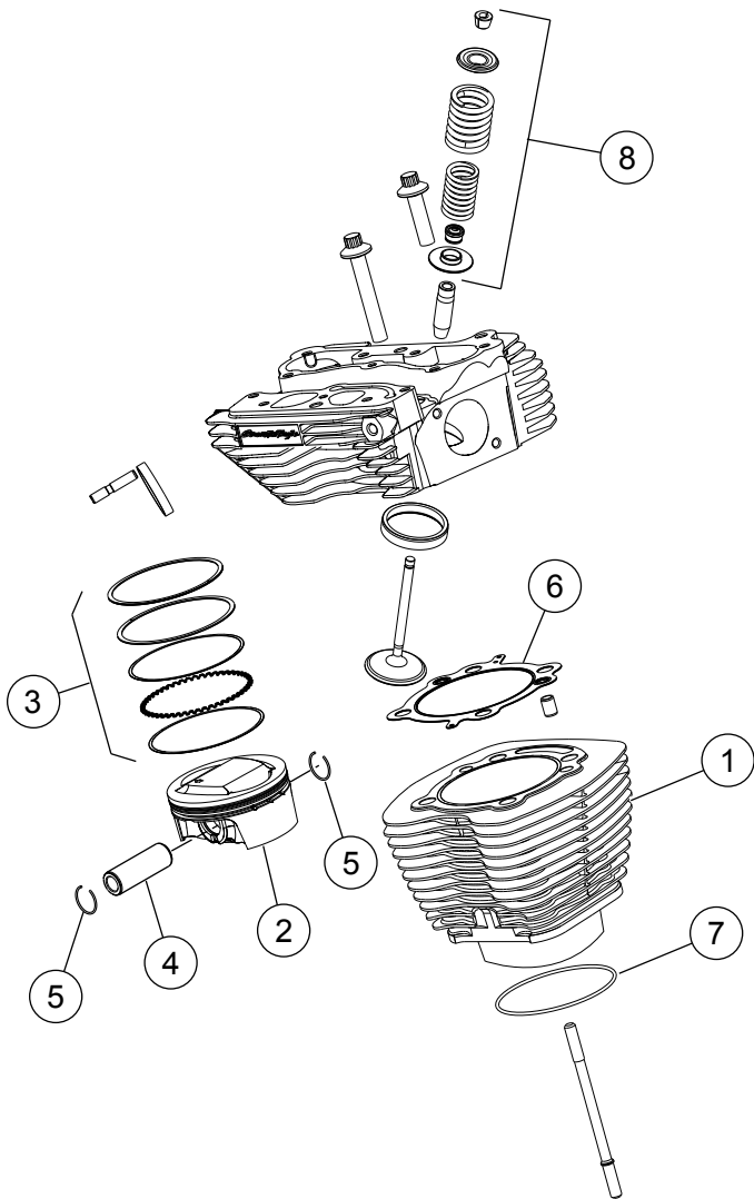
Figura 1. Parti di ricambio: Kit Stage 3 Screamin' Eagle Pro TC 1.690 cm 3 (103 in 3 )
