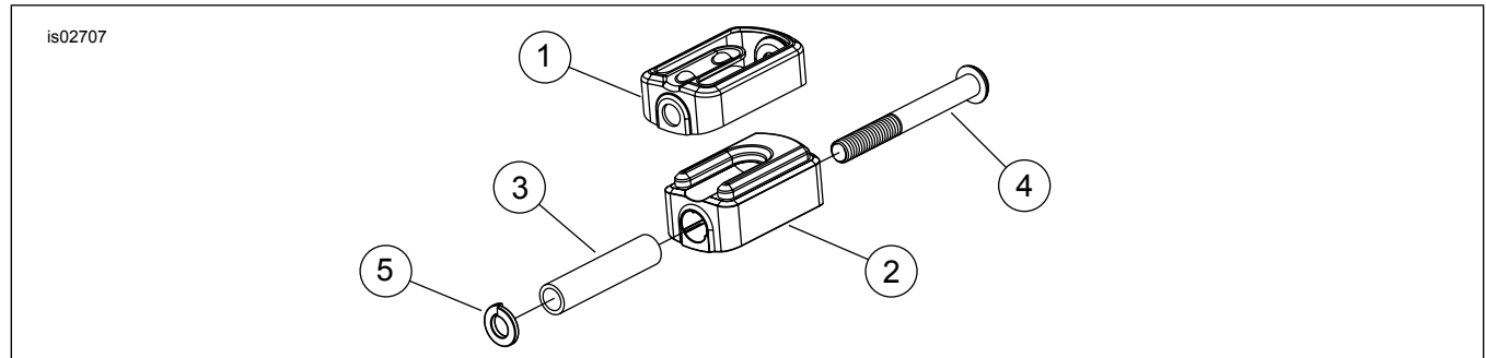
Figure 1. Pièces détachées : kit de pédale de sélection de vitesse Ironside
