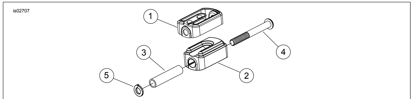
Abbildung 1. Ersatzteile: Ironside Schaltstangenzapfensatz
