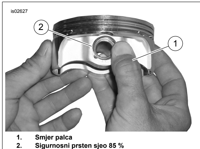
Slika 3. Postavljanje sigurnosnog prstena (prikazani generički klip)
