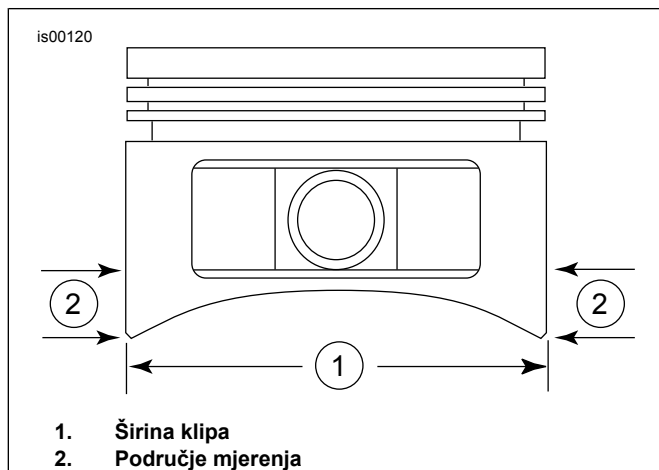
Slika 1. Mjerenja klipa
