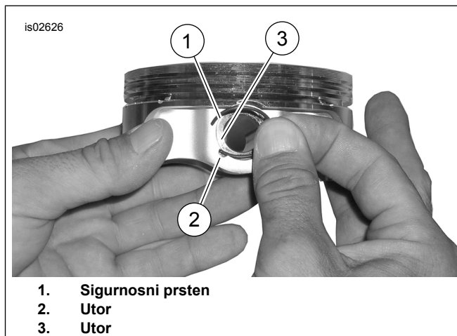
Slika 2. Sigurnosni prsten i klip (prikazani generički klip)
